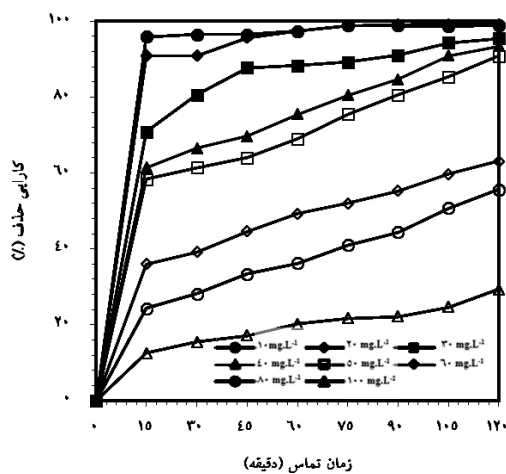
نمودار 3: تأثیر غلظت اولیه‌ی فسفات بر کارایی حذف آن ( \text{pH} = 3 )، مقدار اولیه‌ی نانوکامپوزیت برابر با 0.5 \text{ gL}^{-1}
